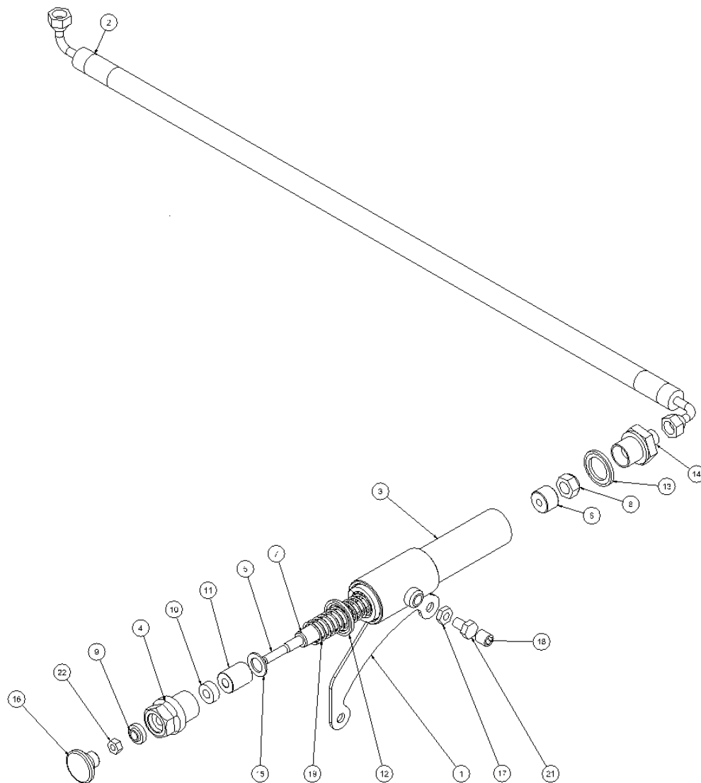
Рис. 4 POD system
